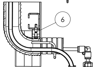
SECTION B-B SCALE 1 : 3
